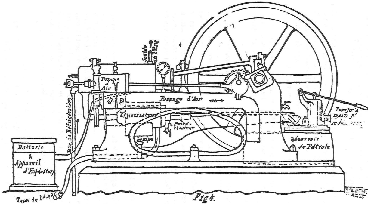
Doorsnee van een petroleummotor.
